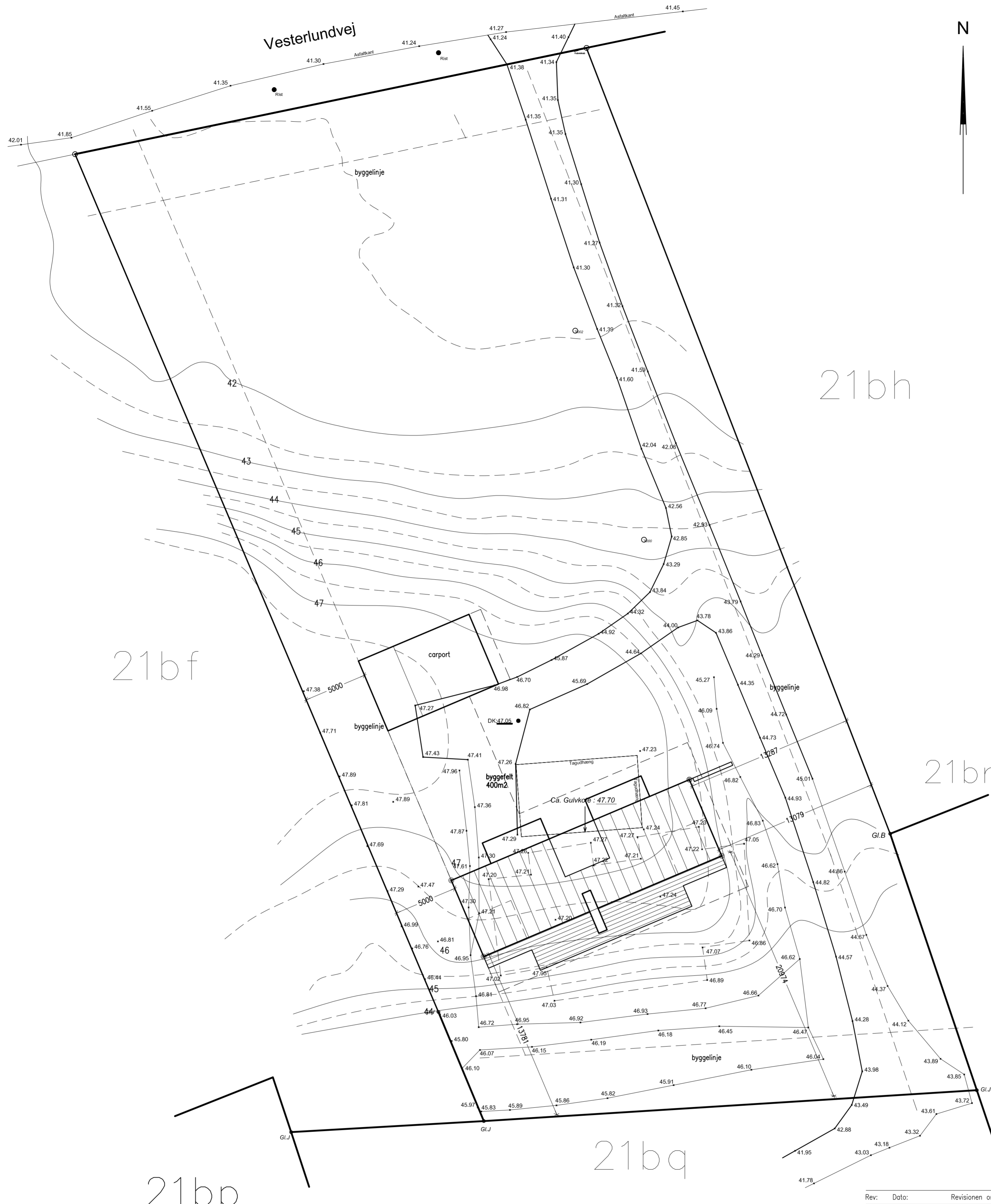
F2 SITUATIONSPLAN 1:200
